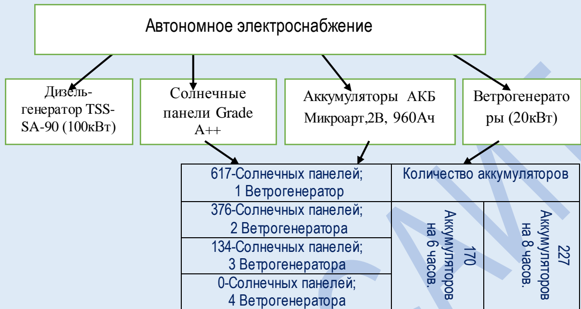
Рисунок 2 – Схема автономного электроснабжения
