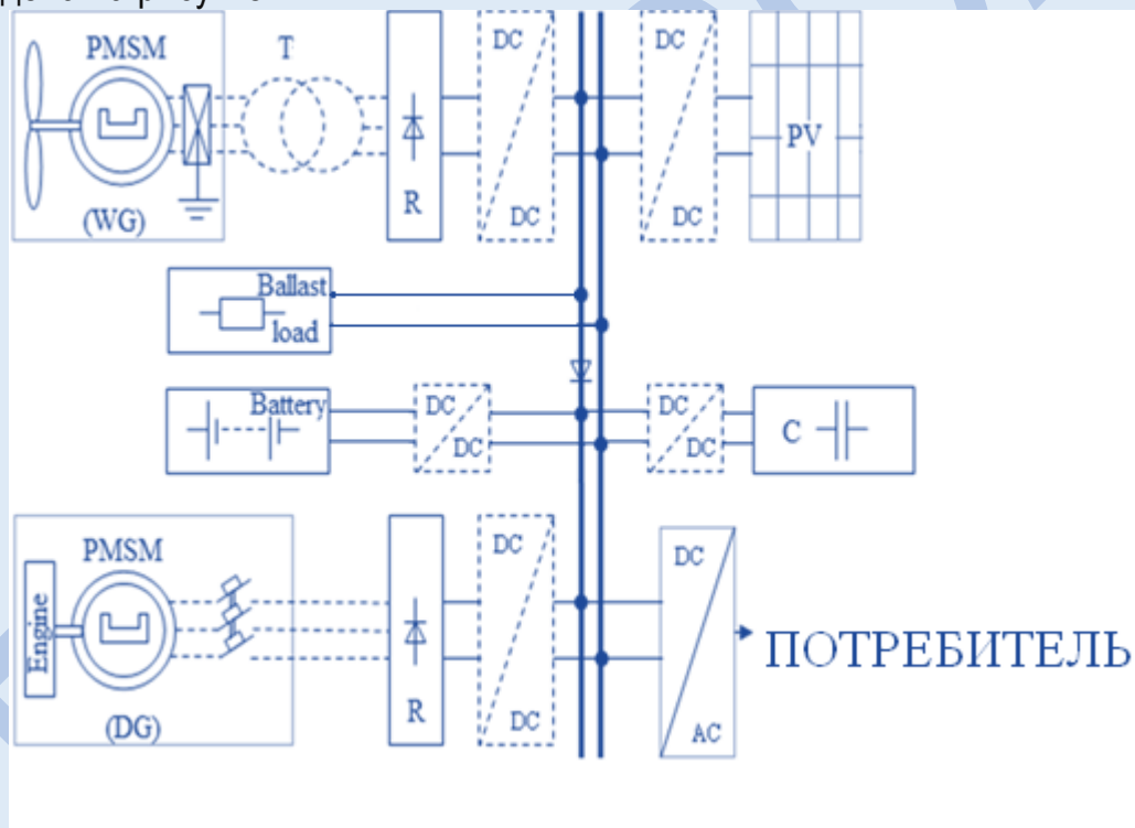
Рисунок 1 - Схема автономной системы электроснабжения на основе возобновляемых источников энергии: WG – ветрогенератор; DG – дизель-генератор; Т – трансформатор; PMSM – синхронный генератор с постоянными магнитами; pV – фотоэлектрический преобразователь; R – выпрямитель; SC – система конденсаторов; DC/DC – преобразователь постоянного тока; DC/AC – инвертор.
